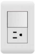
CB-1GY1CA(M) 10AX 127V~1gang 1way switch(M) 15A 127V~1gang socket(M)
